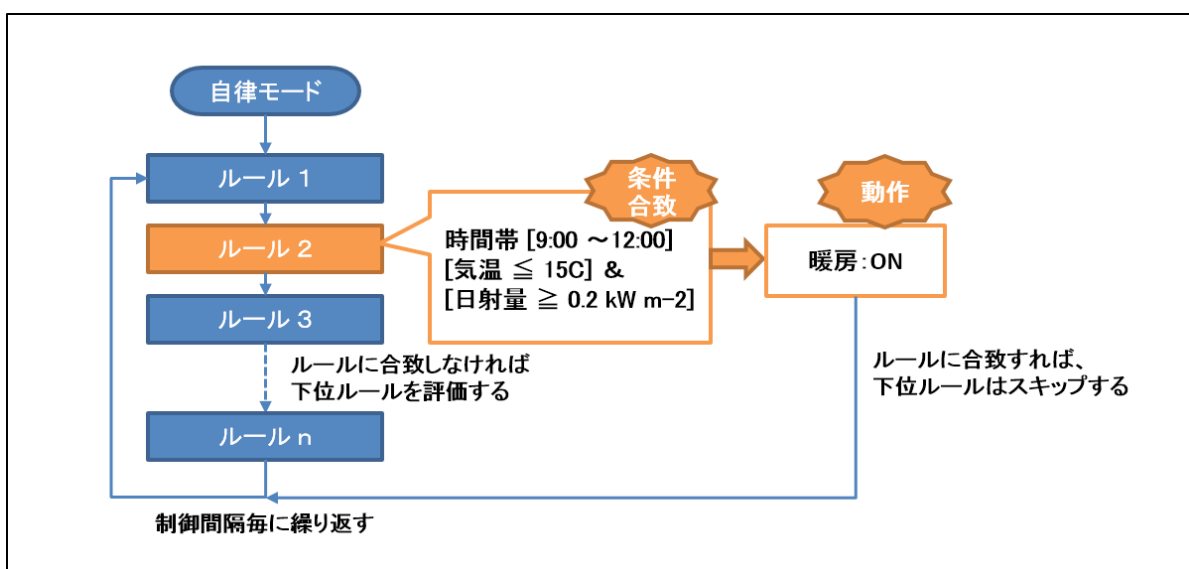
図 28：ルールベース制御概念図
