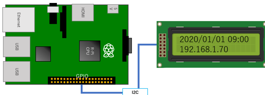
図 62：LCD デバイス接続模式図
