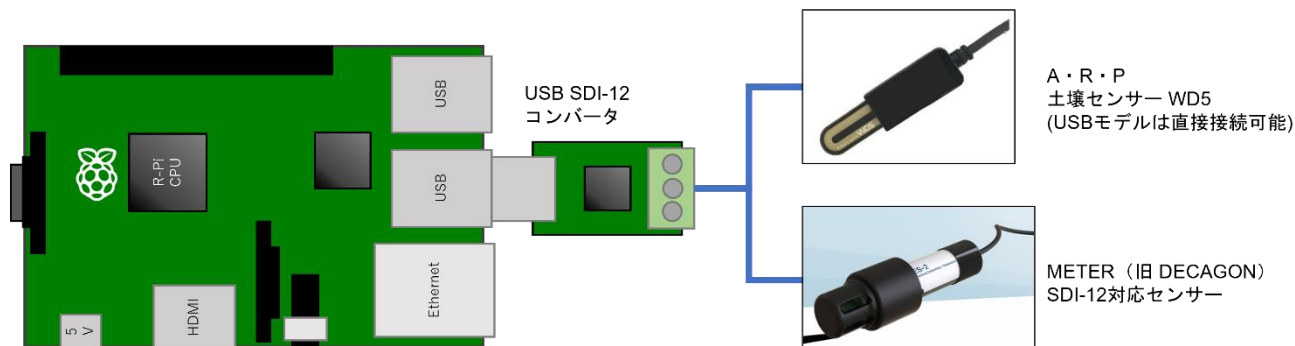
図 60：SDI-12 デバイス接続模式図
