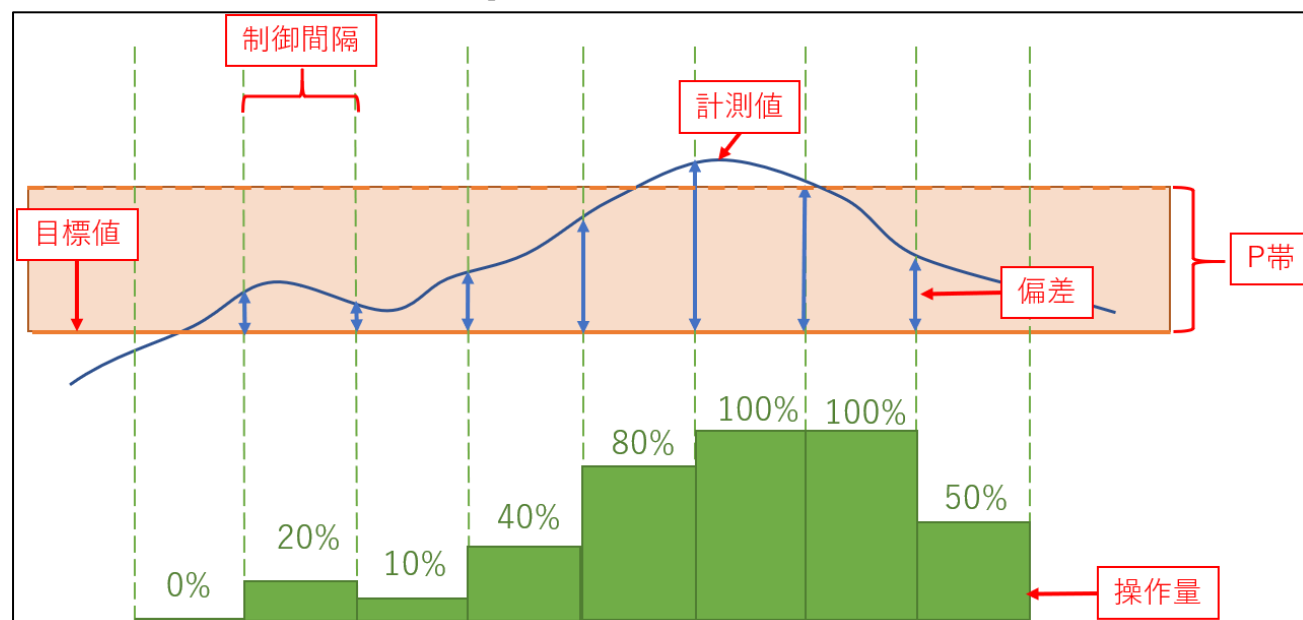
図 33 : P 比例動作イメージ
