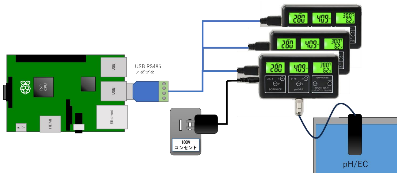
図 50 : Yieryi 3178 接続模式図
