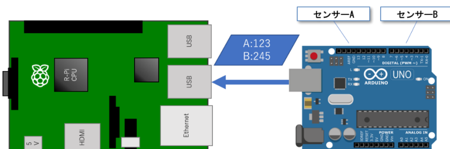
図 58: 汎用シリアル入力デバイス接続模式図
