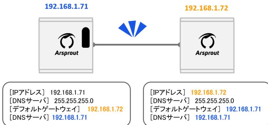
例)ノード同士をLANケーブルで接続する
