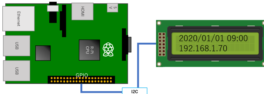
図 62：LCD デバイス接続模式図
