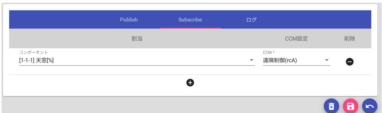
図 15：Subscribe 設定
