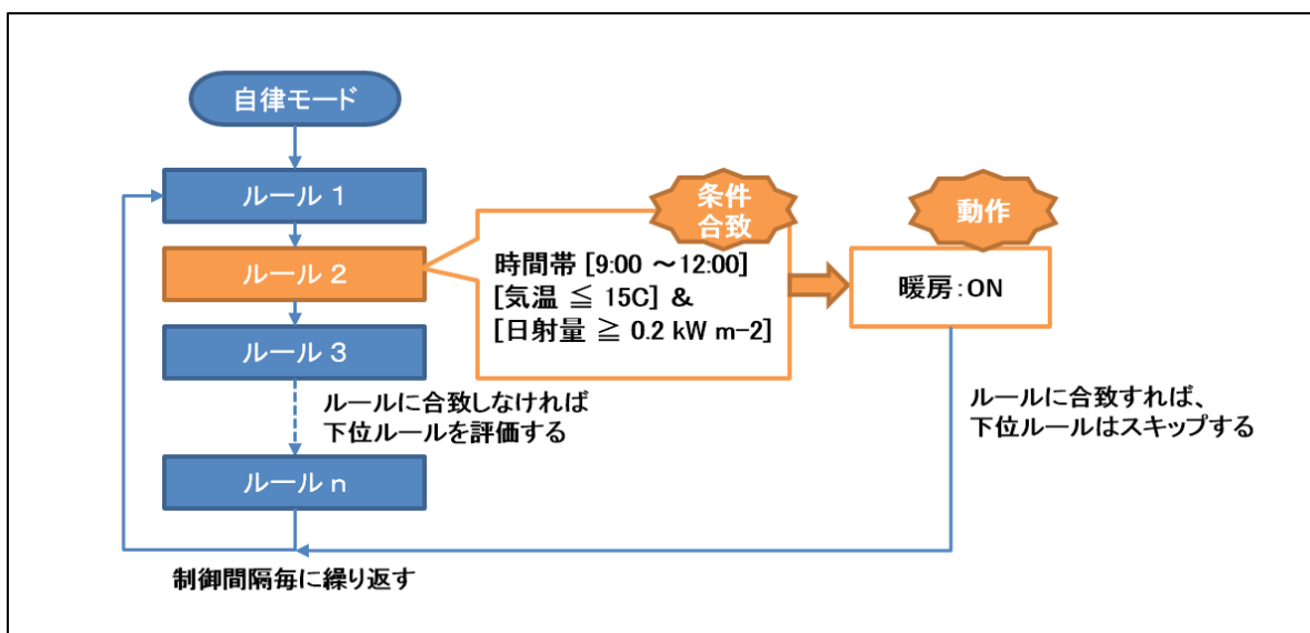
図 29：ルールベース制御概念図
