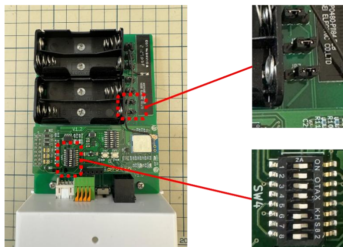
図 4：Air ノード基板（親機）SW4/ジャンパプラグ
