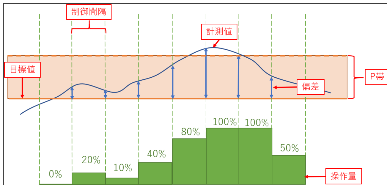
図 32 : P 比例動作イメージ
