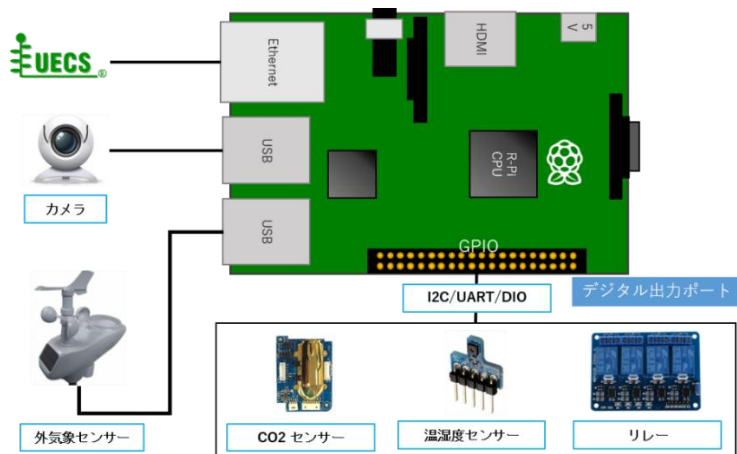
図 40：デバイス接続模式図
