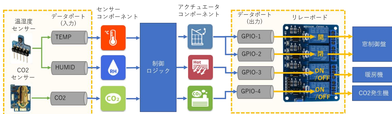
図 41：デバイス機能関連図
