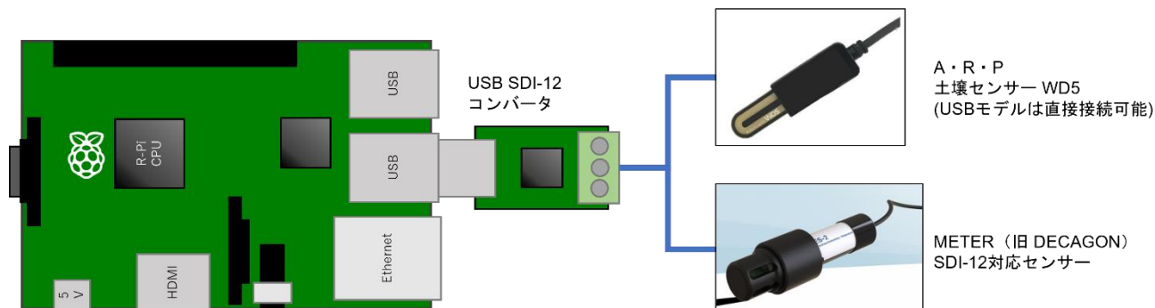
図 59：SDI-12 デバイス接続模式図
