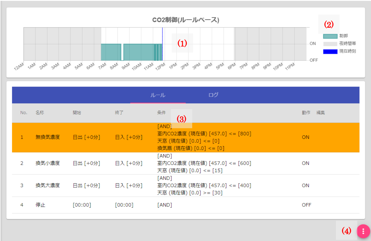
図 29：ルールベース制御モニター画面
