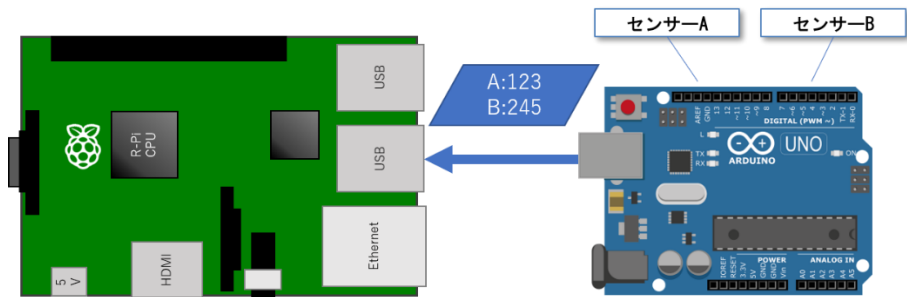
図 57：汎用シリアル入力デバイス接続模式図
