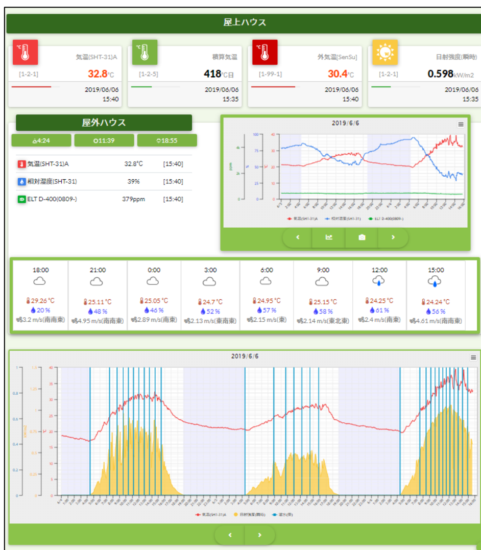
図 71：クラウドサービス画面
