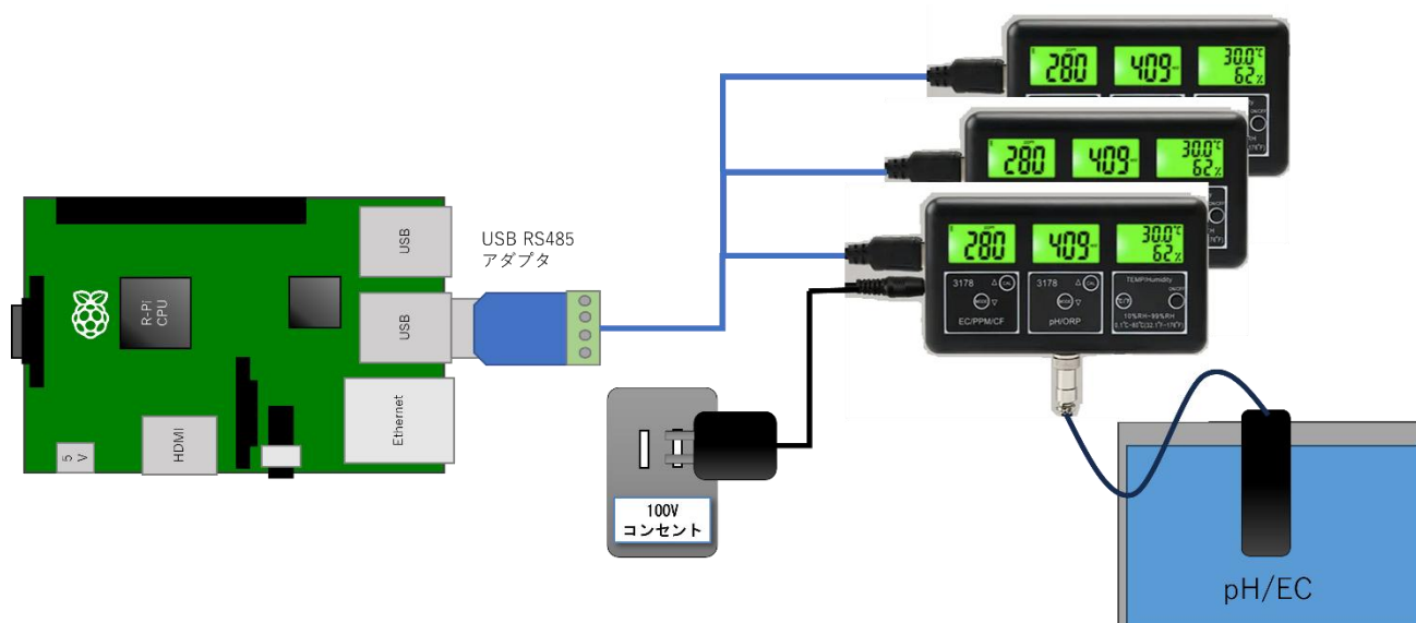
図 49：Yieryi 3178 接続模式図
