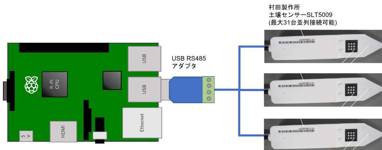
図 46 : SLT5009 接続模式図
