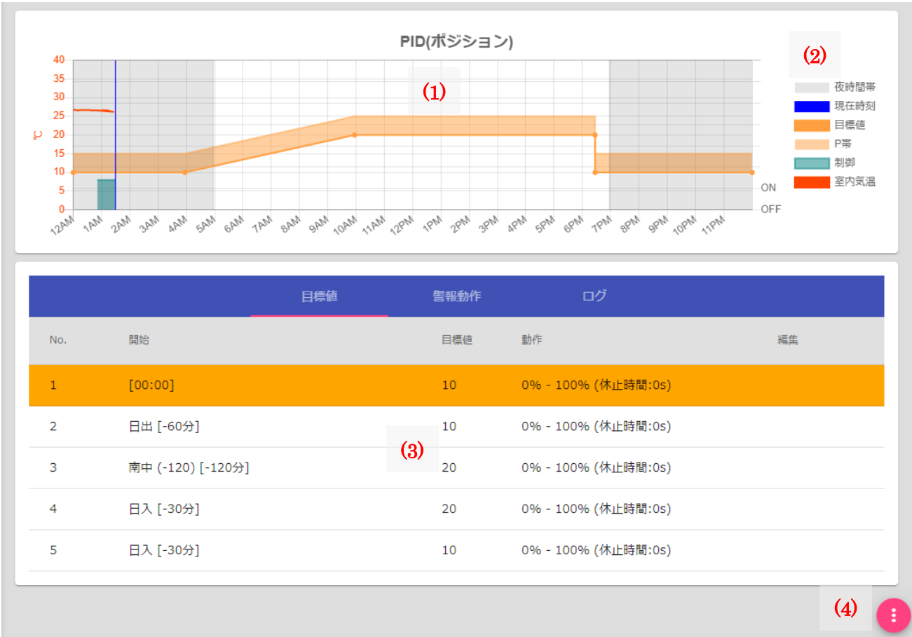
図 33：PID 制御モニター画面
